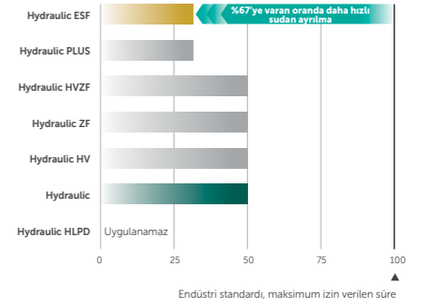
Sudan Ayrılabilirlik Testi Sonuçları (test yöntemi ASTM D1401)
