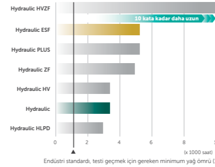
Oksidasyon Stabilitesi Testi Sonuçları (test yöntemi Türbin Yağı Oksidasyon Stabilitesi Testi ASTM D943)
