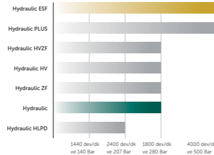
Ürün Performans Seviyesi (pompa hızı ve basıncı)
