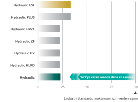
Hidrolik Pompa Aşınma Testi Sonuçları (test yöntemi EATON 35VQ25)
